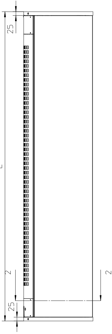
Vorderansicht
